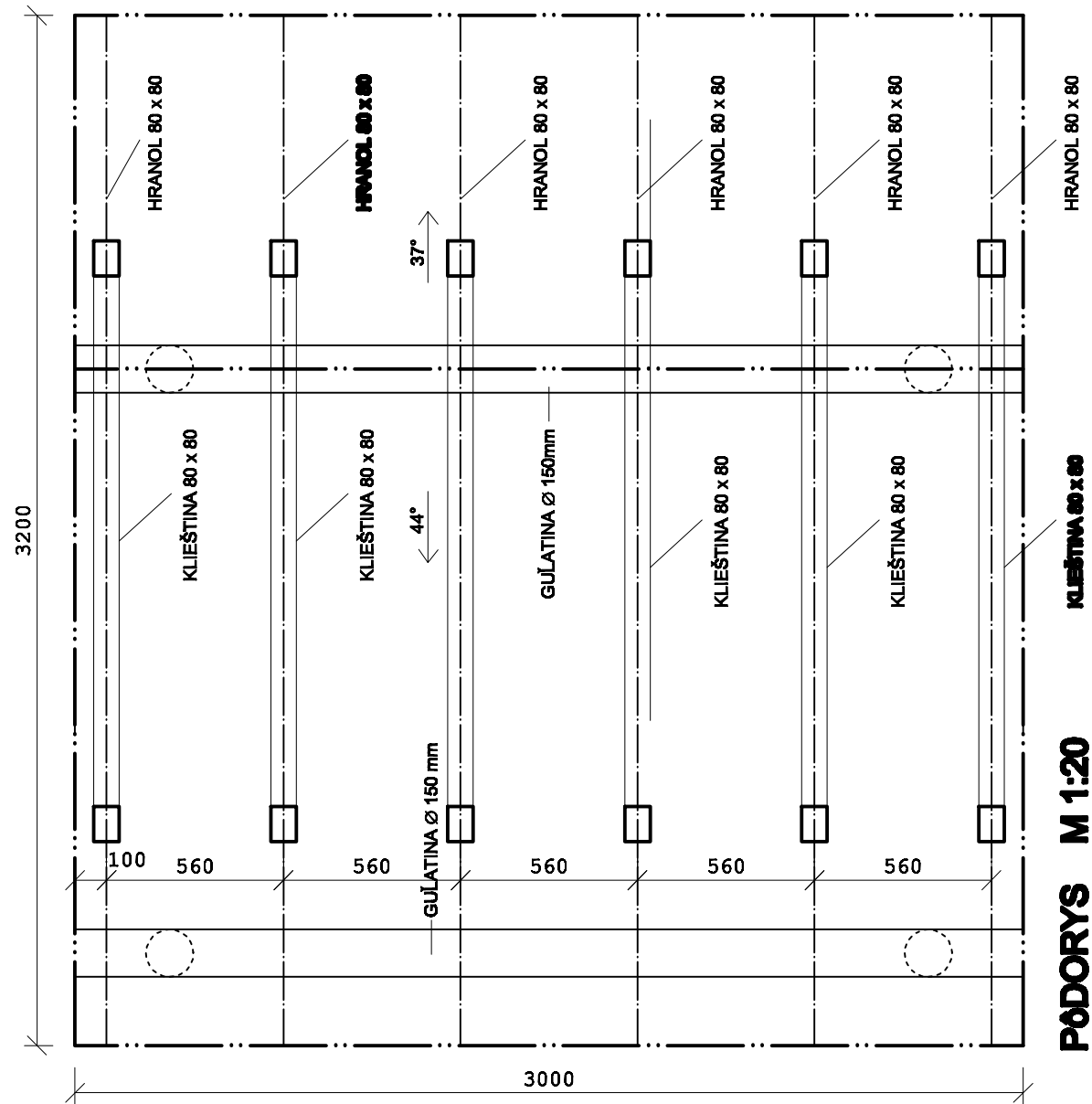
PÔDORYS M 1:20
