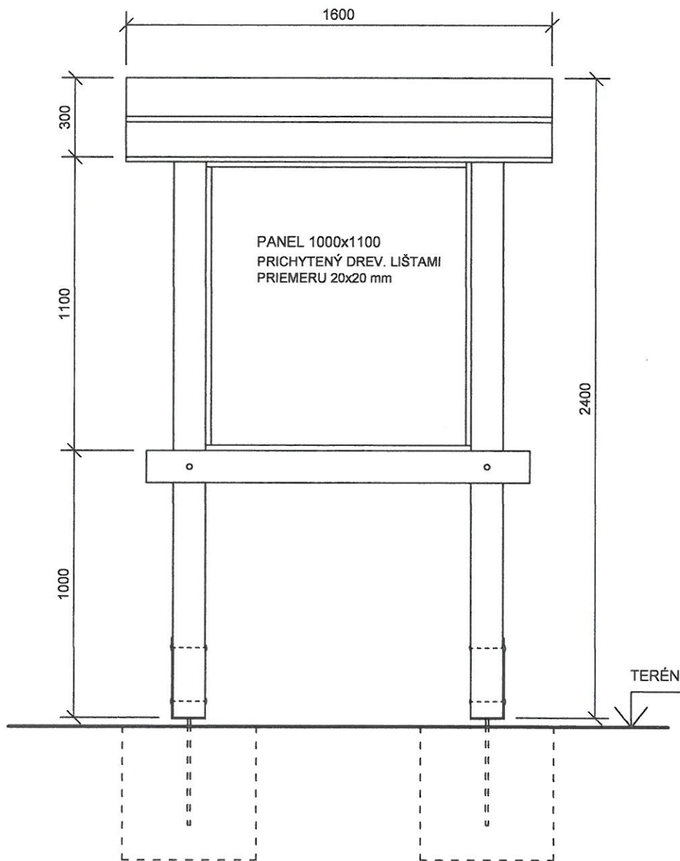
POHLAD ČELNÝ M 1:20
