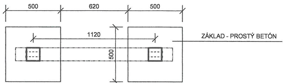
PŮDORYS M 1:20
