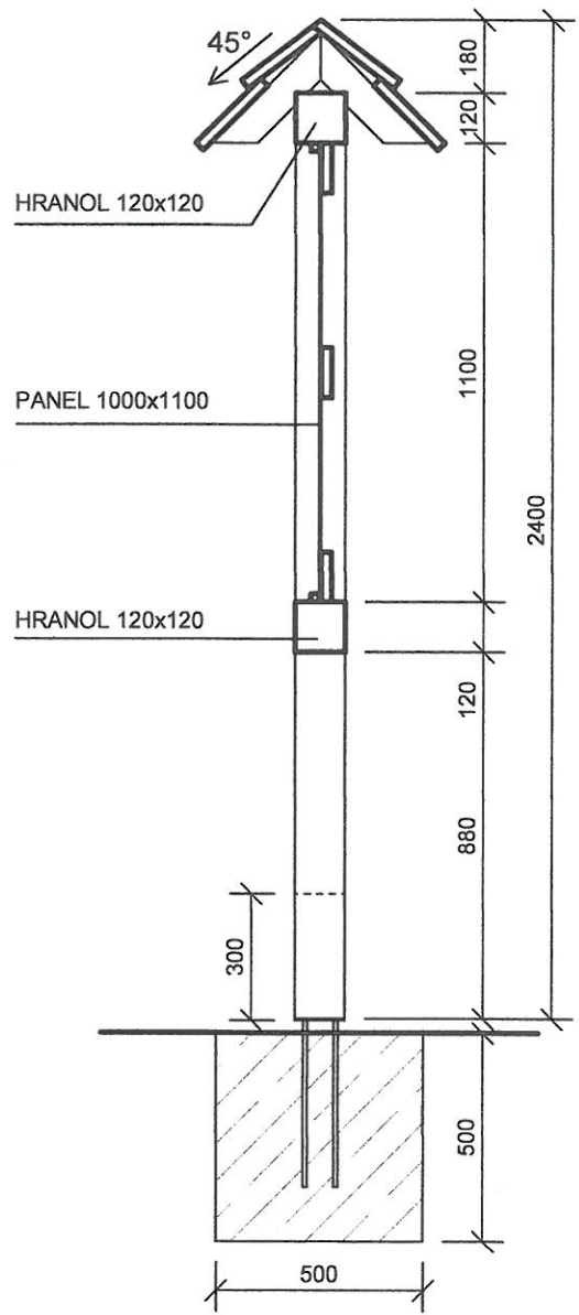
PRIEČNY REZ M 1:20
