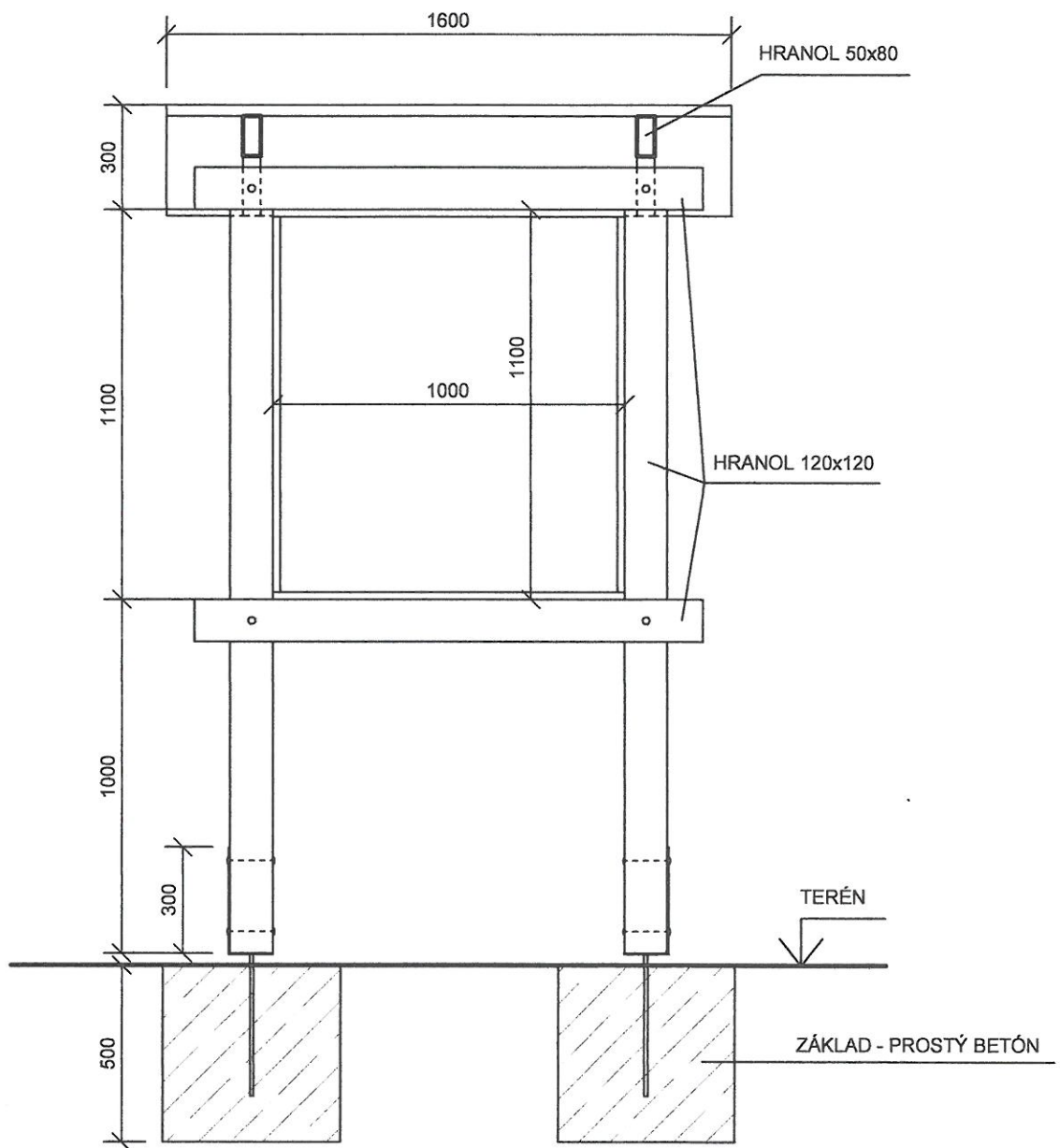
POZDĚŽNY REZ M 1:20
