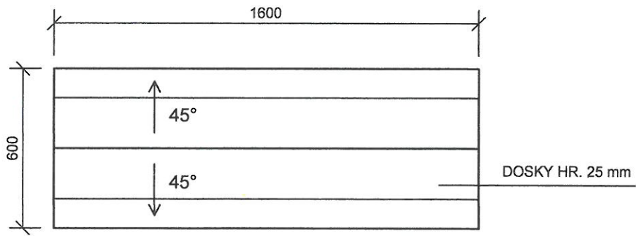
POHLAD NA STRECHU M 1:20
