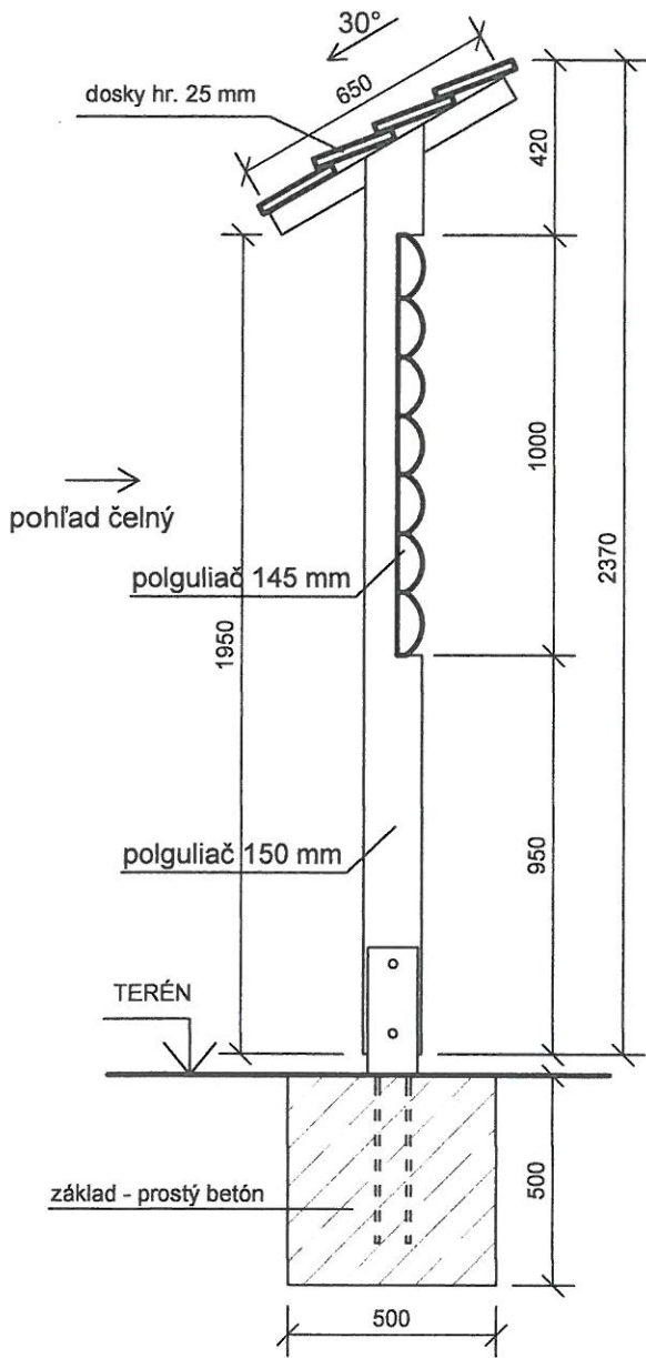
PRIEČNY REZ
