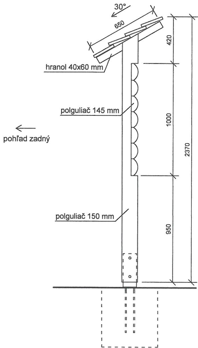
POHL'AD BOČNÝ M 1:20
