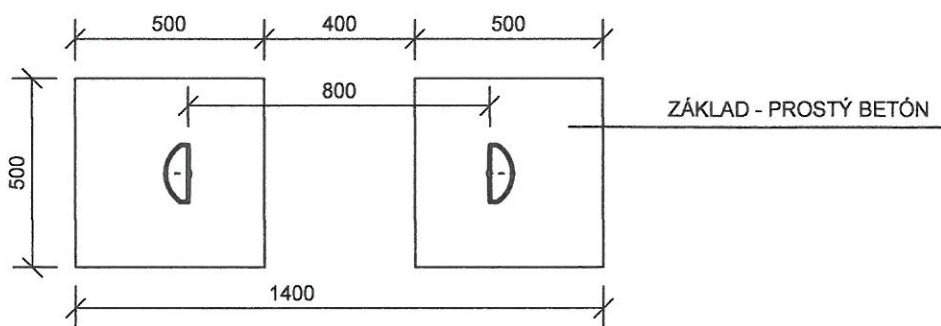
PÓDORYS M 1:20
