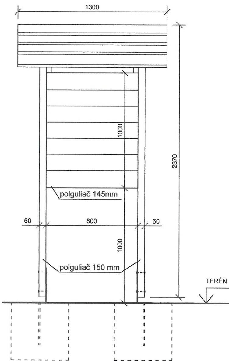
POHĽAD ČELNÝ M 1:20
