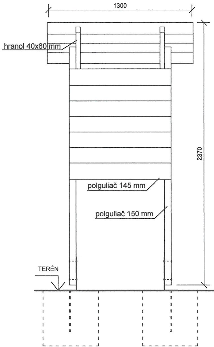
POHĽAD ZO ZADU M 1:20
