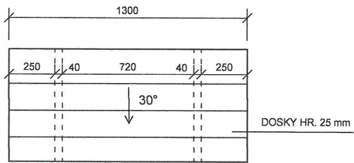
POHĽAD NA STRECHU M 1:20
