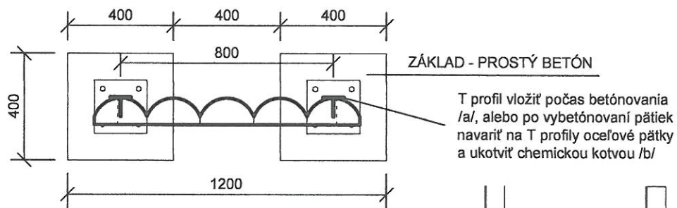
PÔDORYS M 1:20
