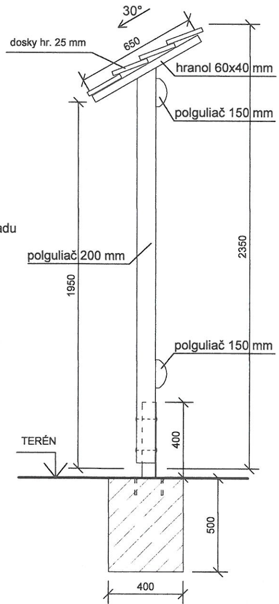
POHĽAD BOČNÝ M 1:20
