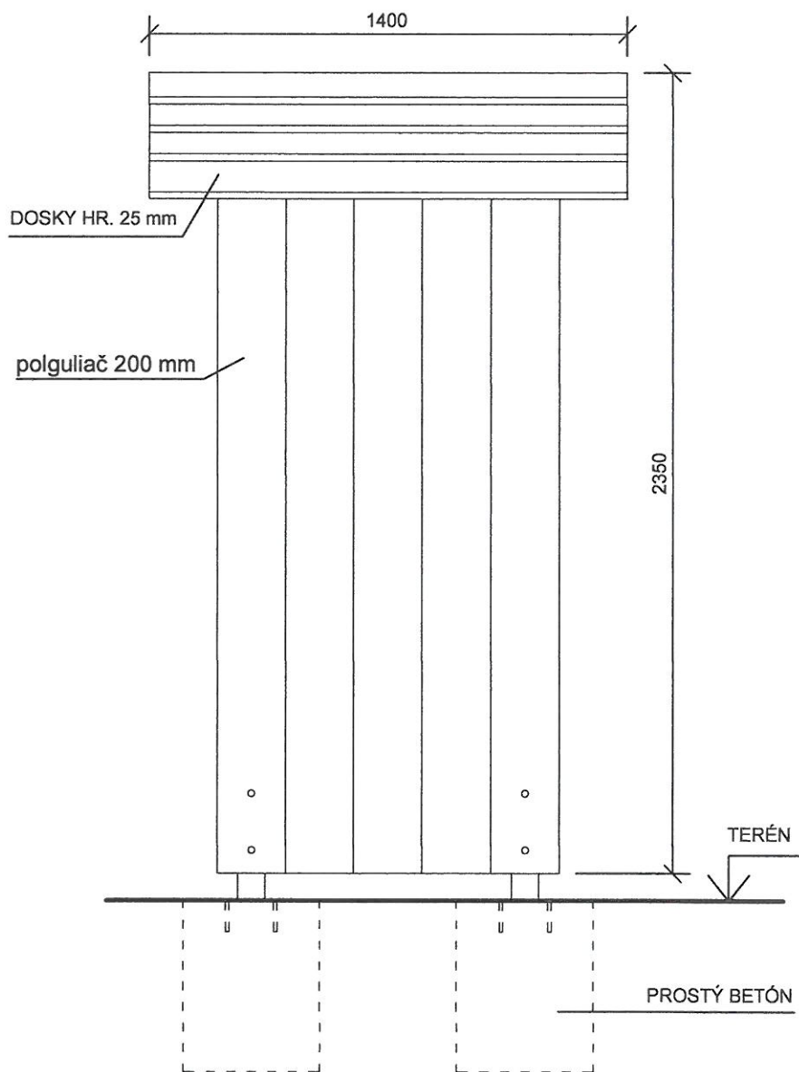
POHĽAD ČELNÝ M 1:20
