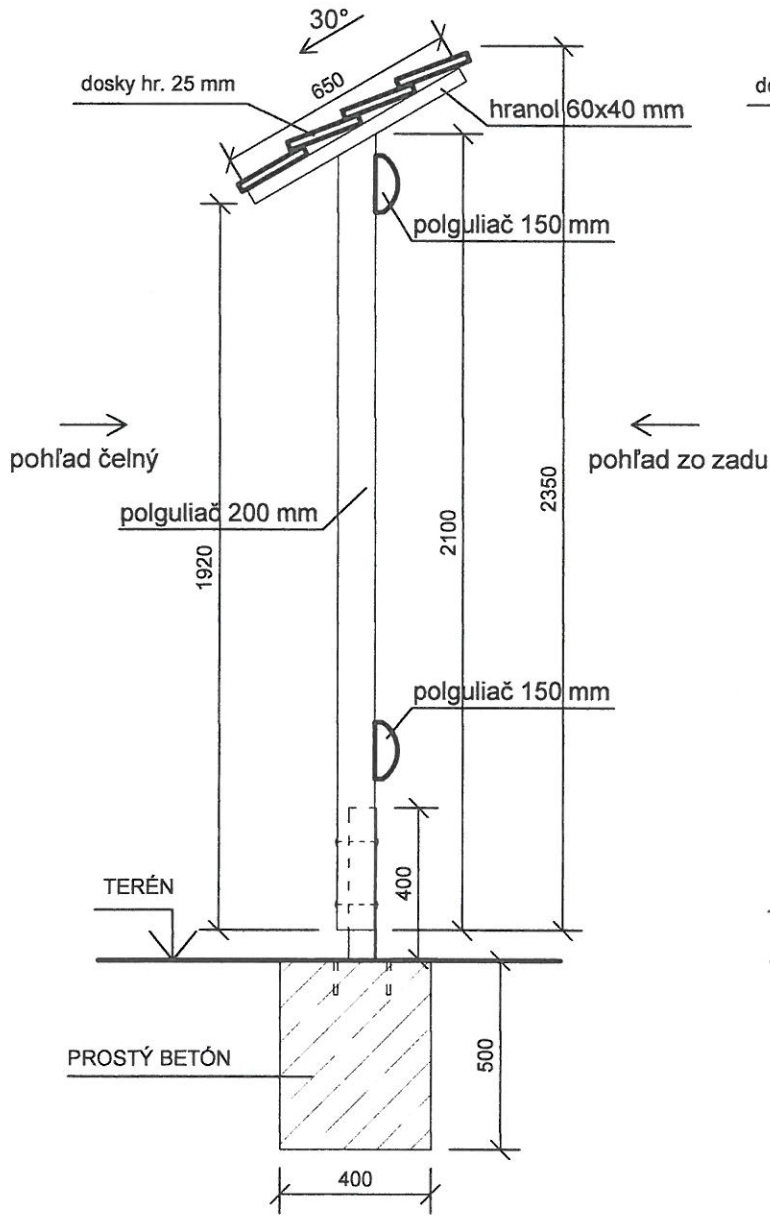
PRIEČNY REZ M 1:20
