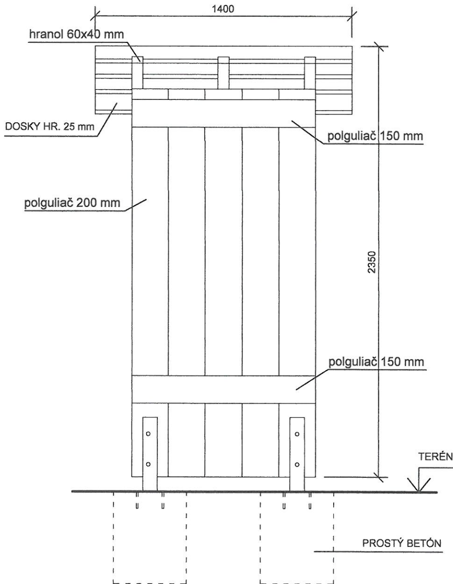
POHĽAD ZO ZADU M 1:20
