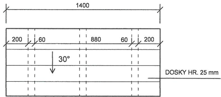
POHĽAD NA STRECHU M 1:20
