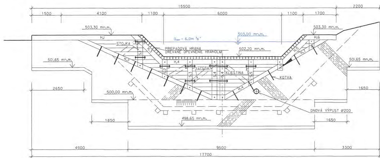
REZ II-II
