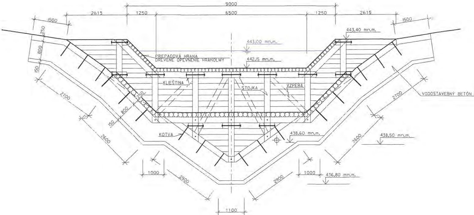
REZ II-II
